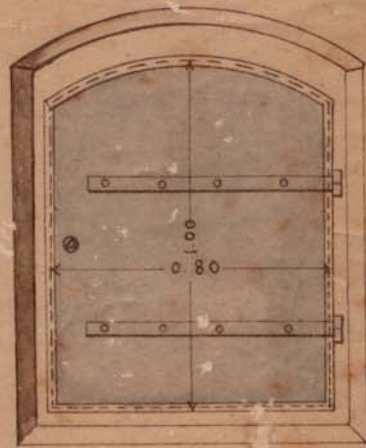
Ansicht
